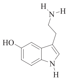
Serotonin; 5-HT
