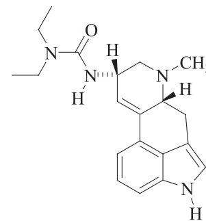
Lisuride
