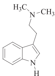
DMT
