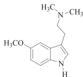
5-Methoxy-DMT
